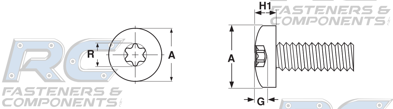
METRIC - SIX-LOBE PAN HEAD DIN 750TX HEAD PER DIN 750CE
